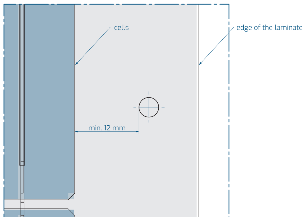
Abb. 3: Mindestabstand nachträglicher Montagebohrungen zu elektrisch leitenden Komponenten
