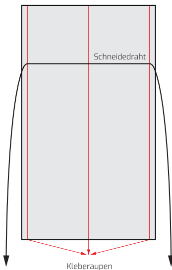
Abb. 11: Demontage von geklebten Modulen mittels Schneiddraht.
