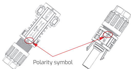
Abb. 7: Kennzeichnung der Polarität auf den PV4-5 Steckverbindern
