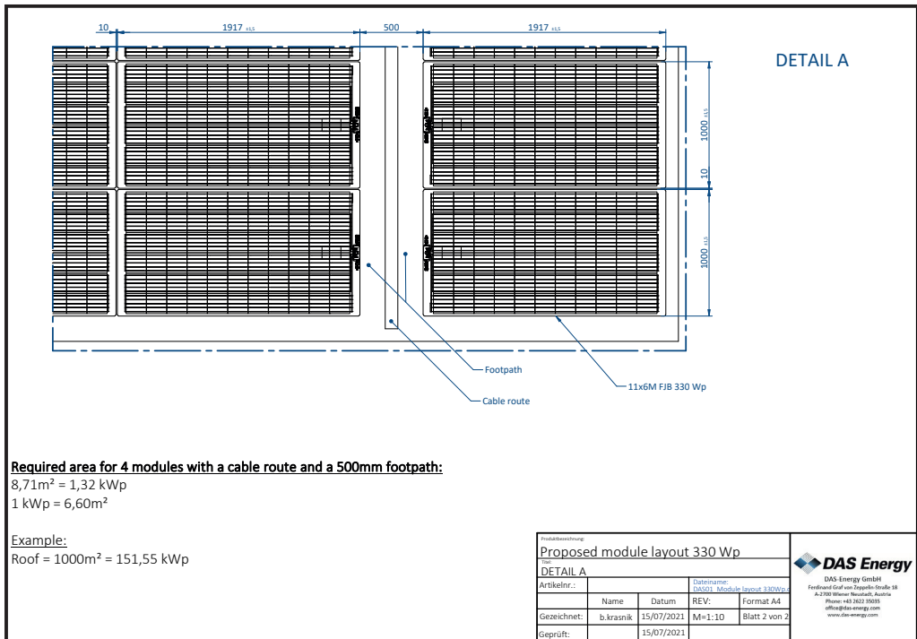
Abb. 2: Beispiel eines typischen Belegungsplanes für Flachdächer (Modultyp 11x6 FJB) – Detailansicht
