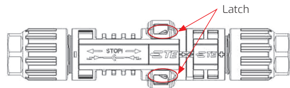
Abb. 8: Zusammenschließen der PV4-5 Steckverbinder
